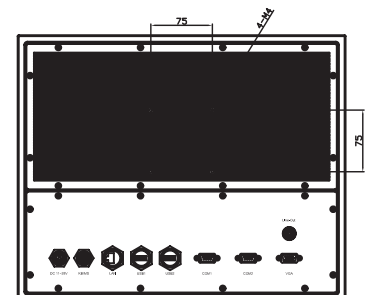
Optional I/O
